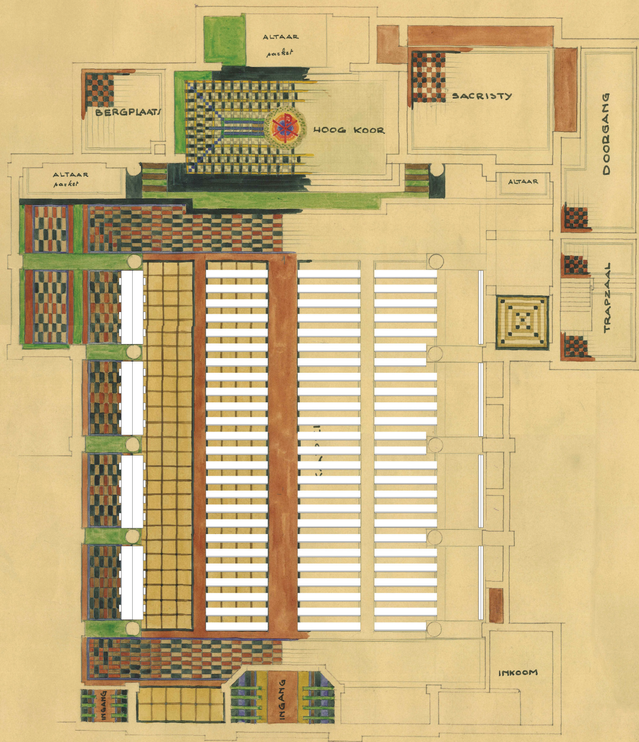
PLAN GELYKVLOERO
